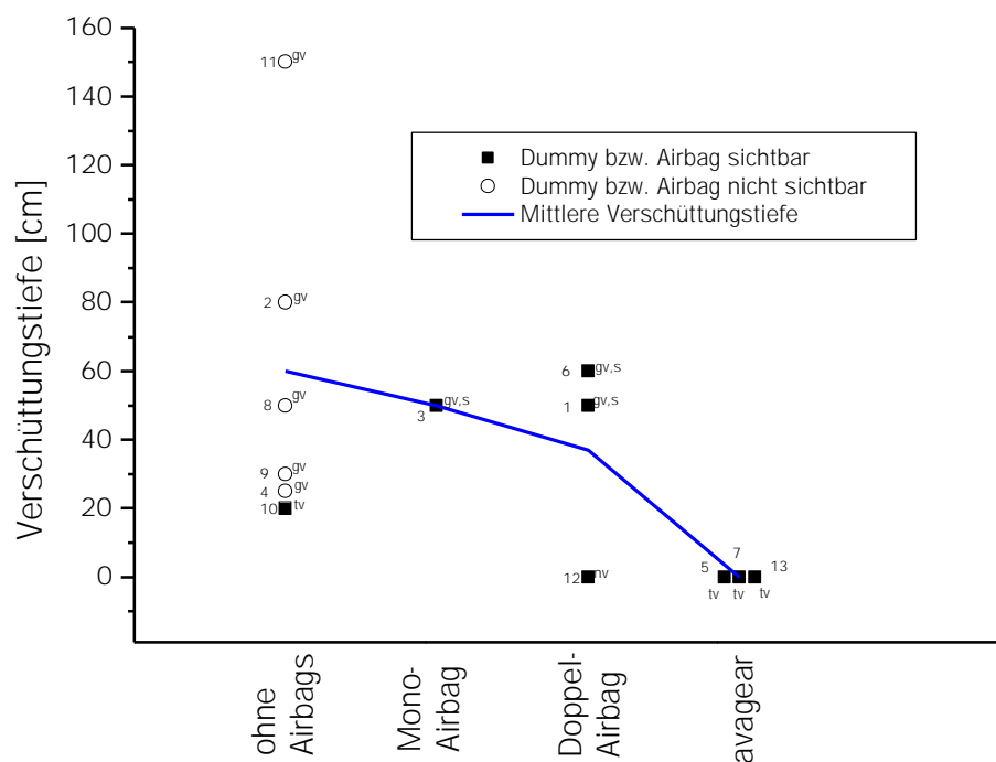
Abb. 7: Verschüttungstiefen der Dummies ohne resp. mit Lawinenairbags.
