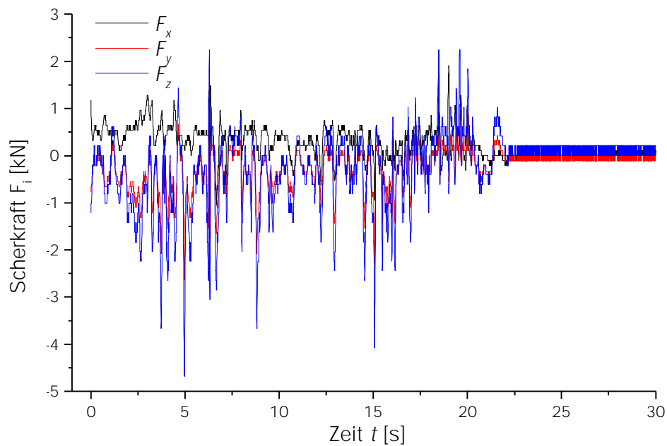
Abb. 8: Zeitserien der Scherkräfte im Halswirbelsäulenbereich des Messdummies mit „avagear“-Airbag.
