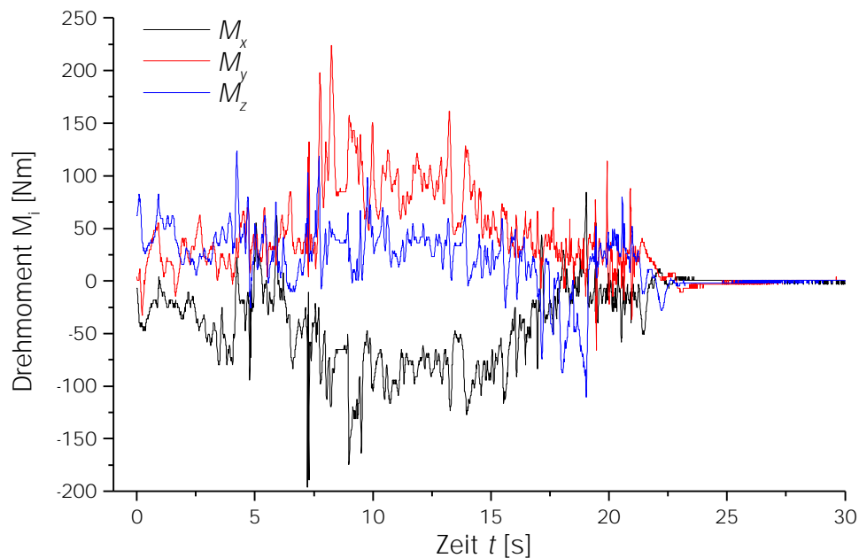
Abb. 9: Zeitserien der Drehmomente im Halswirbelsäulenbereich des Messdummies mit „avagear“-Airbag.
