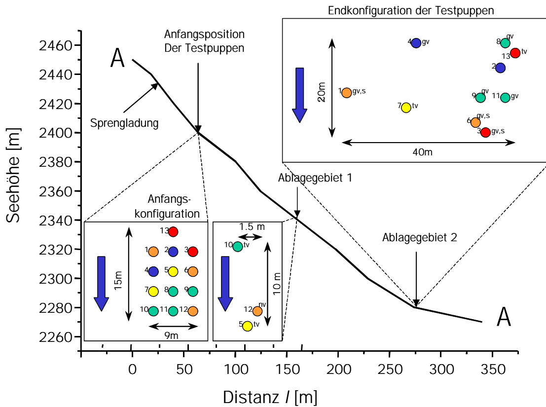
Abb. 5: Profil längs der Linie A-A (Abb. 4) mit Anfangs- und Endpositionen Versuchsdummies. Bezeichnung der Dummies gemäss Tabelle 1.
