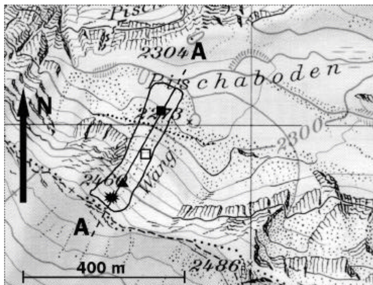
Abb. 4: Versuchshang „Wäng“ im Skigebiet Pischaboden mit Positionen der Sprengladungen (*), Anfangs-(Dreieck) und Endpositionen (Quadrat) der Dummies. Reproduziert mit Bewilligung der Eidg. Landestopographie.
