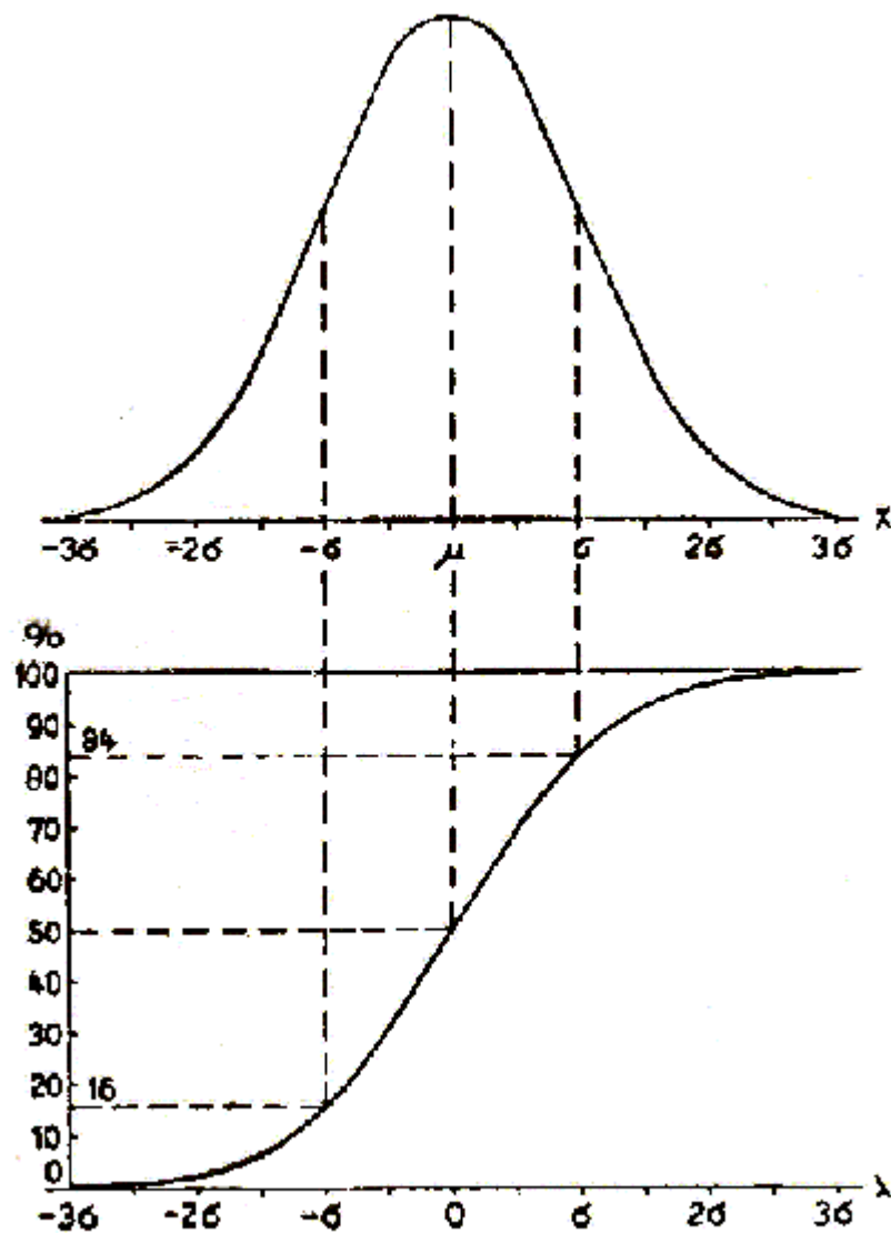
Abb. 47. Gauss-Kurve und Summenprozentkurve.
