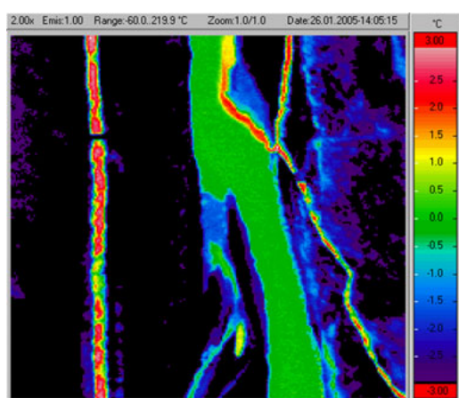
Figure 6.8 : Variabilité de la température dans l'élargissement de la Thur à Schaffäuli TG/ZH. En haut : photographie en lumière naturelle. En bas : photographie infra-rouges (résolution : 1 m 2 ; précision : 0,1 °C), janvier 2005 (Photos : C. Tanner, EMPA ; U. Uehlinger, Eawag).
